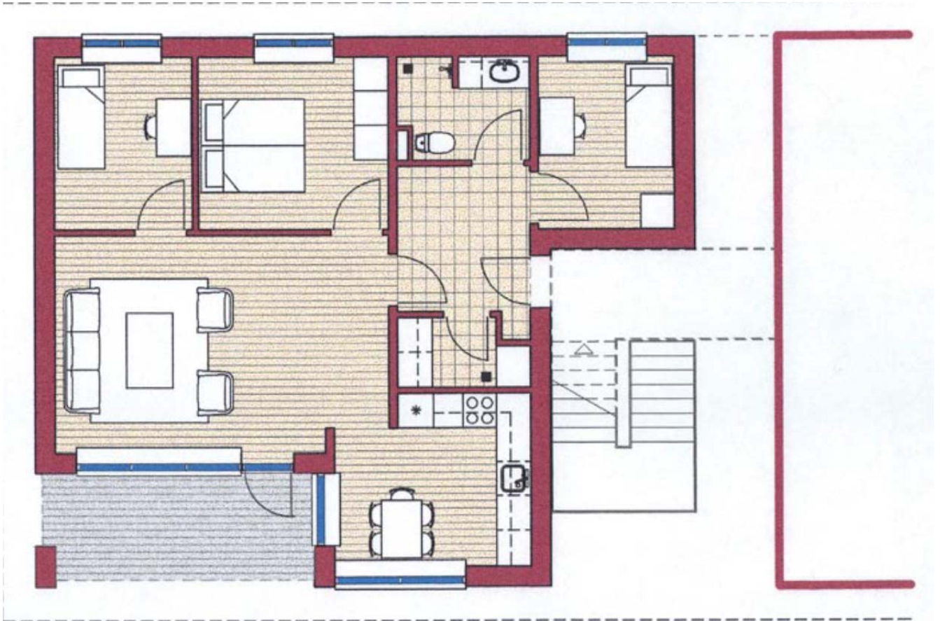
Boligtype A Stueplan 89 kvm. + udhus Terrasse og have
