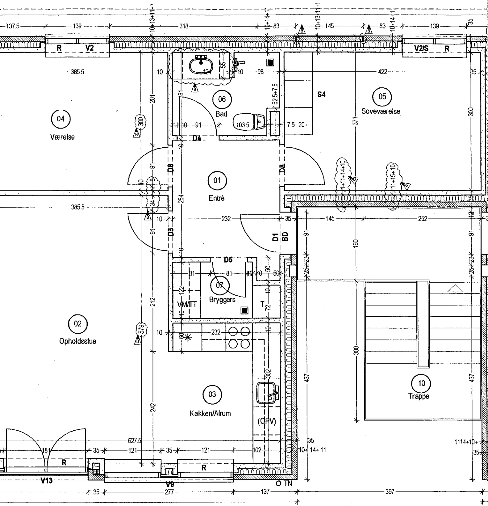
Lejlighed / type D
